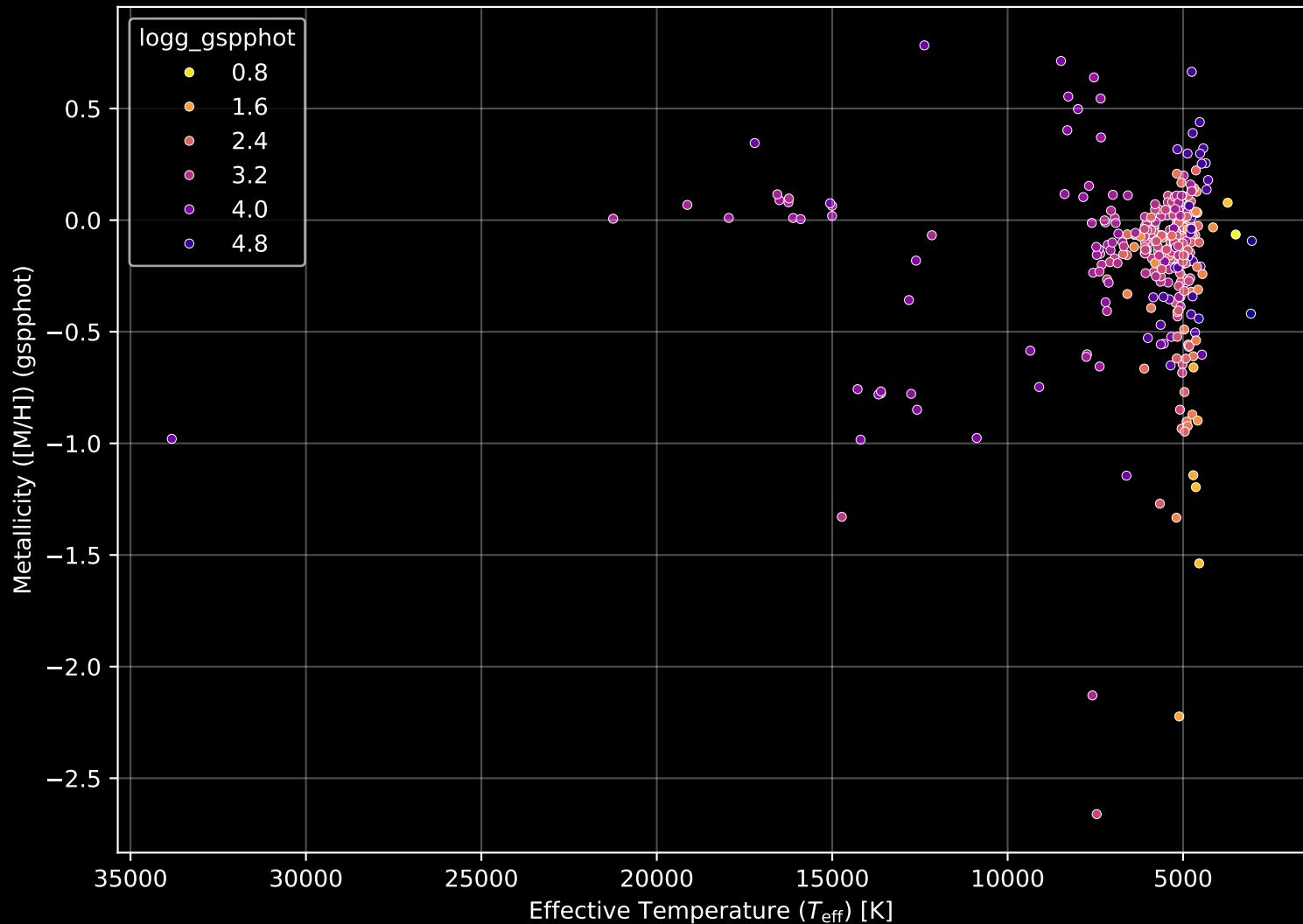
APOGEE DR17 Field: [173+00] Stellar Population Parameters (n= 331)
